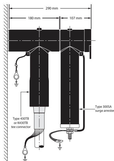
300PB – SA Surge Arrestor
